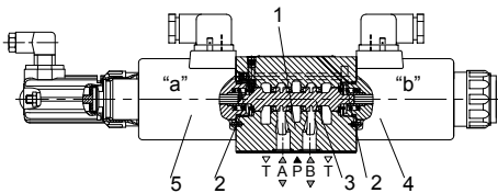
Type 4WRE 10...-L2X/...
