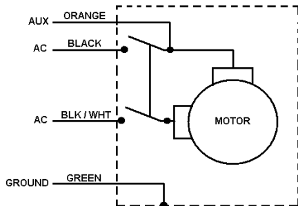
230 VOLT WIRING DIAGRAM
